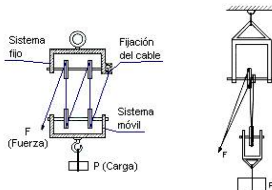
Fig. 1: Mecanismo diferencial Fig. 2: Aparejo diferencial
