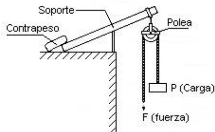
Fig. 5: Garrucha
