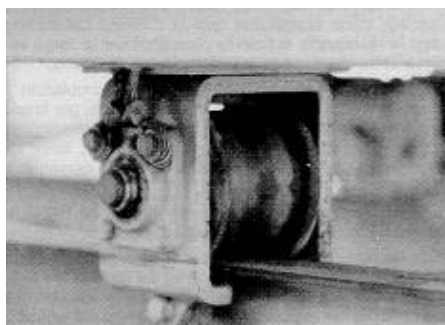
Fig. 9: Raíl en doble T y grapa antivuelco en rueda de carretilla
