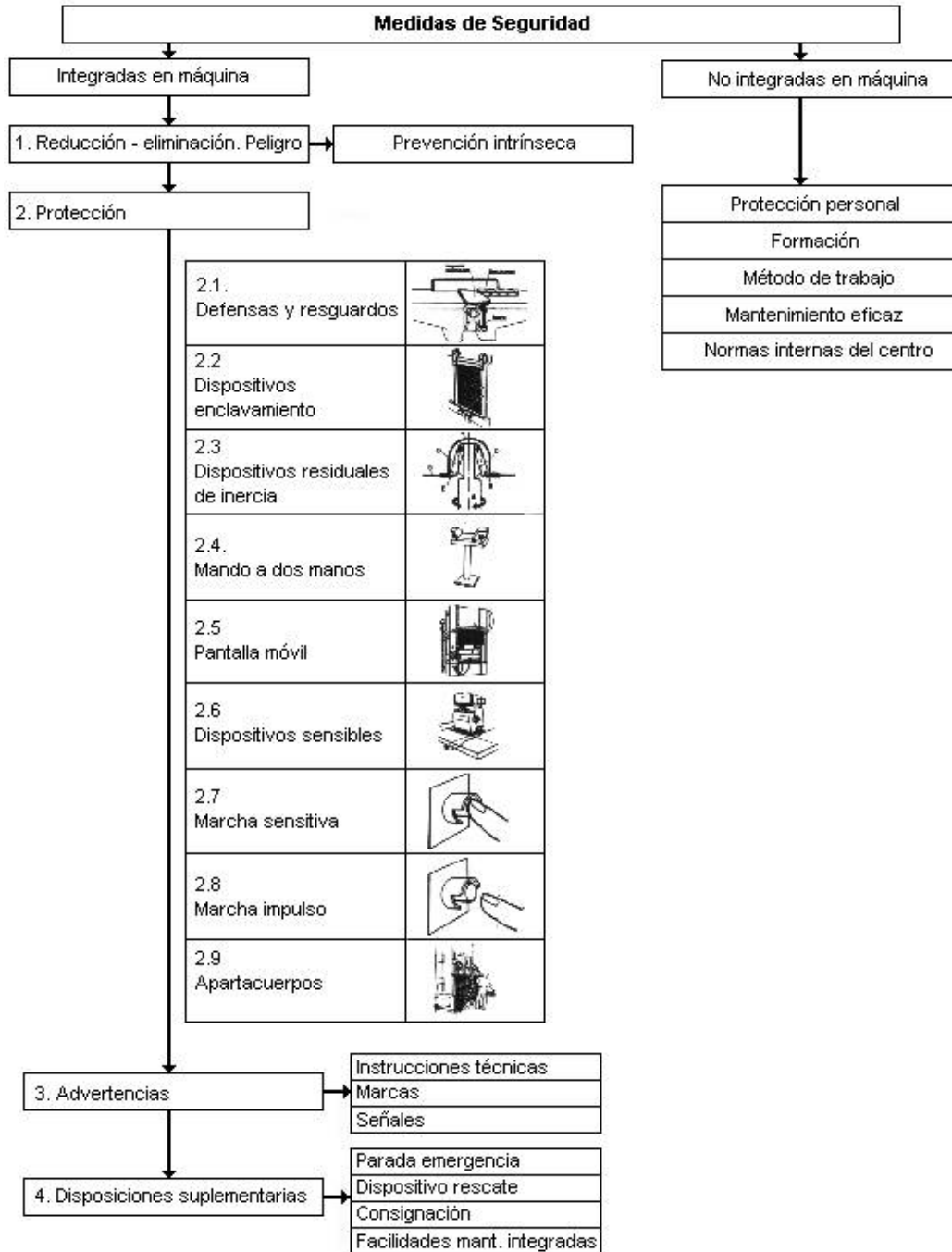
Fig. 2: Medidas de seguridad en máquinas
