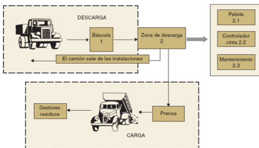
Figura 1 Proceso de un centro de transferencia de residuos
